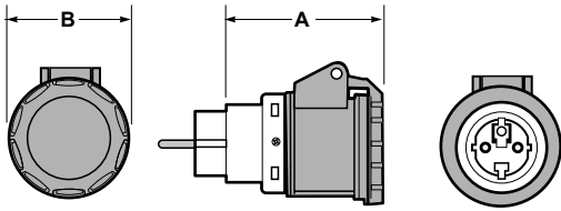
Adaptador doméstico-industrial IP20 / Domestic-industrial IP20
